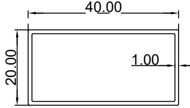
مستطيل (1*20*40) ملم الرقم التسلسلي للصنف: FG40X20X1 الوزن (Kg/m): 0.316
