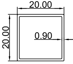
مربع (0.9*20*20) ملم الرقم التسلسلي للصنف: FG20X20X0.9A الوزن (Kg/m): 0.187
