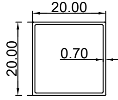
مربع (0.7*20*20) ملم الرقم التسلسلي للصنف: XE0202 الوزن (Kg/m): 0.147
