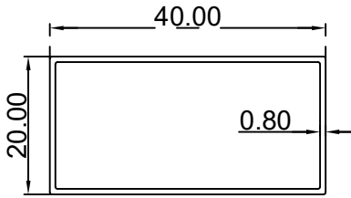
مستطيل (0.8*20*40) ملم الرقم التسلسلي للصنف: BLT3581 الوزن (Kg/m): 0.256
