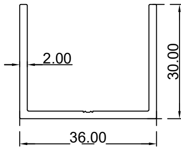
شبرتس قاطع الرقم التسلسلي للصنف: BLT3576 الوزن 0.499:(Kg/m)
