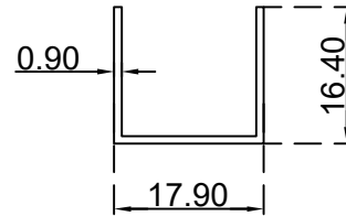
شبرتس مستطيل 20 ملم الرقم التسلسلي للصنف: C17.9X16.4X0.9 الوزن 0.118:(Kg/m)
