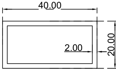
مستطيل (2*20*40) ملم الرقم التسلسلي للصنف: FG40X20X2C الوزن (Kg/m): 0.609
