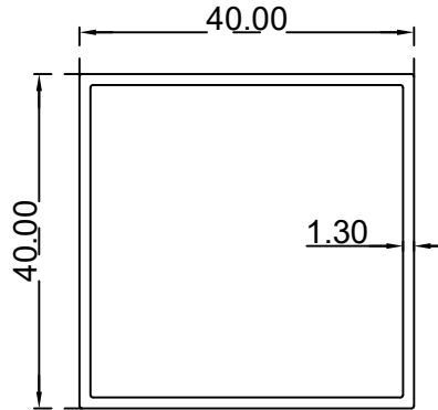
مربع (1.3*40*40) ملم الرقم التسلسلي للصنف: FG40X40X1.3A الوزن (Kg/m): 0.547
