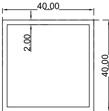
مربع (2*40*40) ملم الرقم التسلسلي للصنف: G40X40X2 الوزن (Kg/m): 0.824
